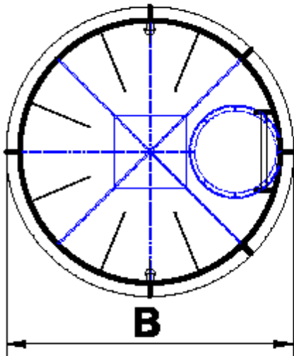
vodorovný řez
