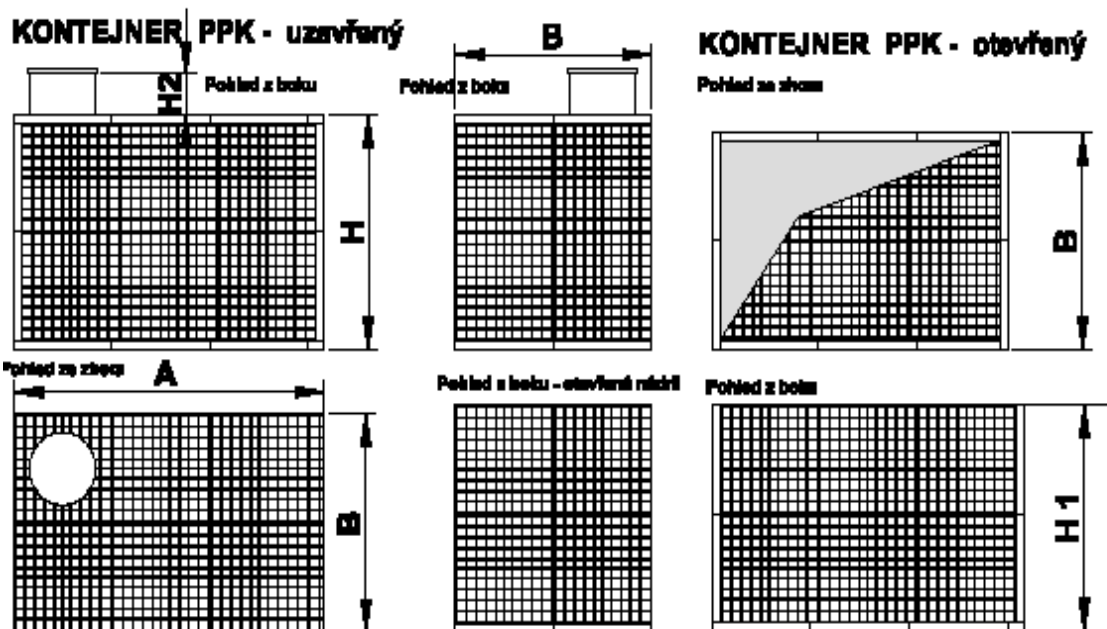
STANDARTNÍ ROZMĚRY PLASTOVÝCH NÁDRŽÍ,
