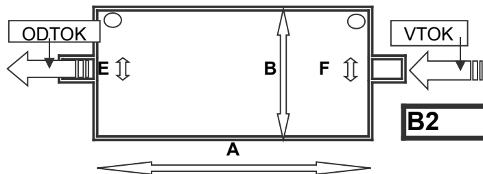
SCHEMA NAPOJENÍ BZF12,16,20
